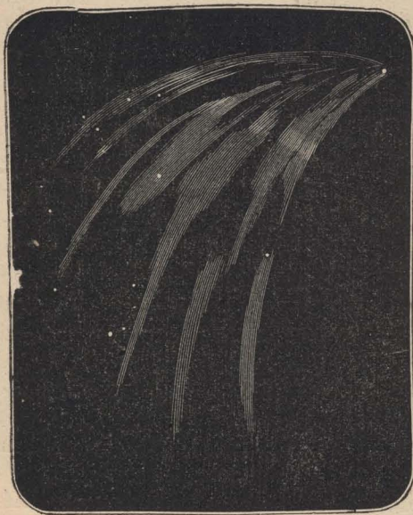
Cometa de cola partida.
